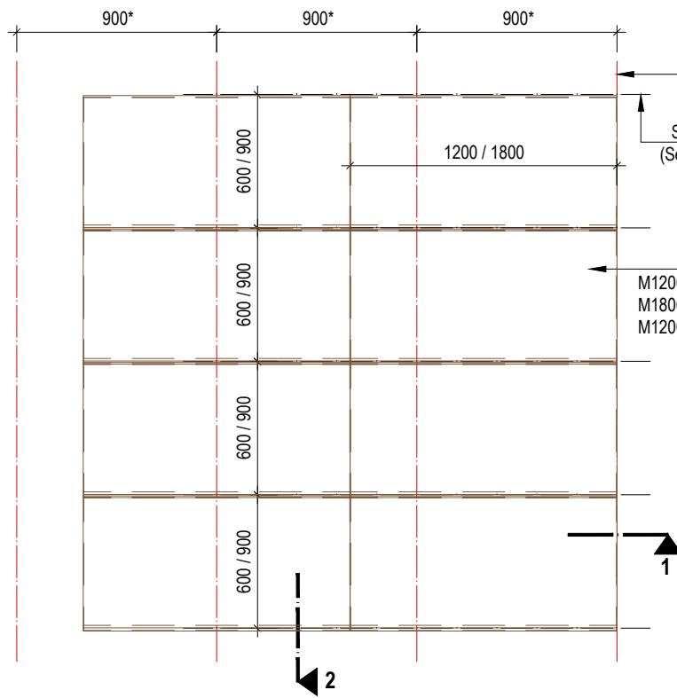
TILE LAY-OUT scale 1:30
