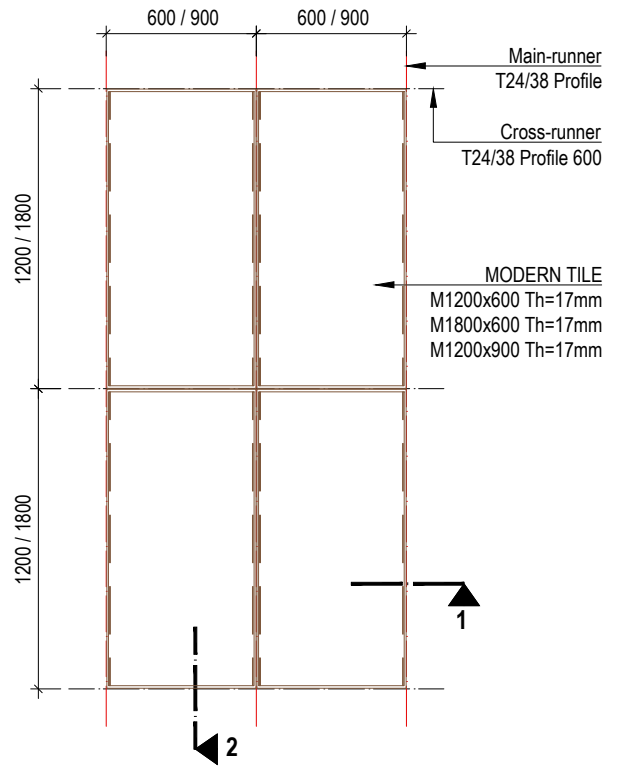
TILE LAY-OUT scale
